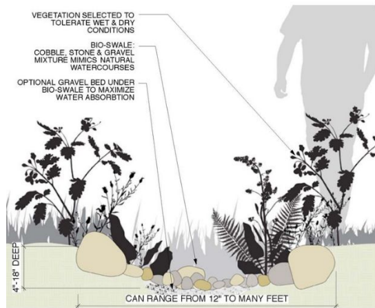
Swales
